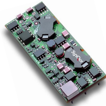
PQ60012EML15 Module
